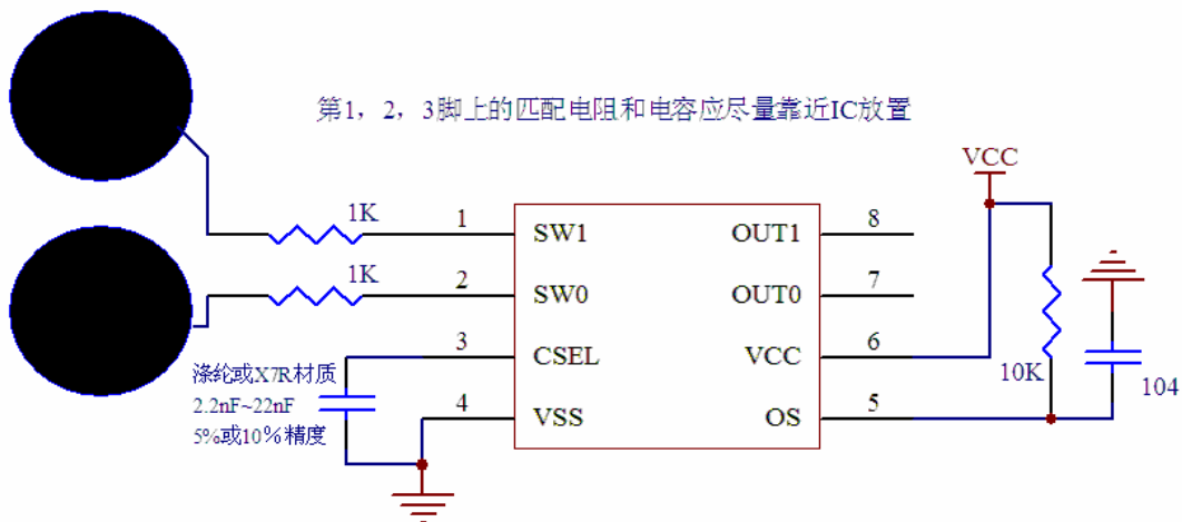
图 4: WTC02SP 应用原理图
