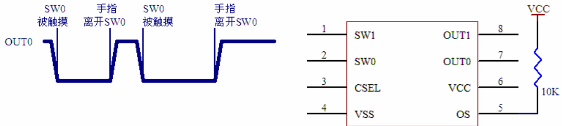
图 2: WTC02SP OS 接 VCC 时按键输出时序图
