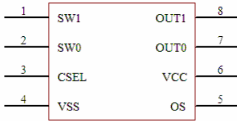
图 1: WTC02SP 引脚图
